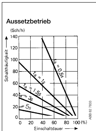
Schalzhäufigkeit in Abhängigkeit von der relativen Einschaltdauer ED in %, t_a : Motoranlaufzeit
